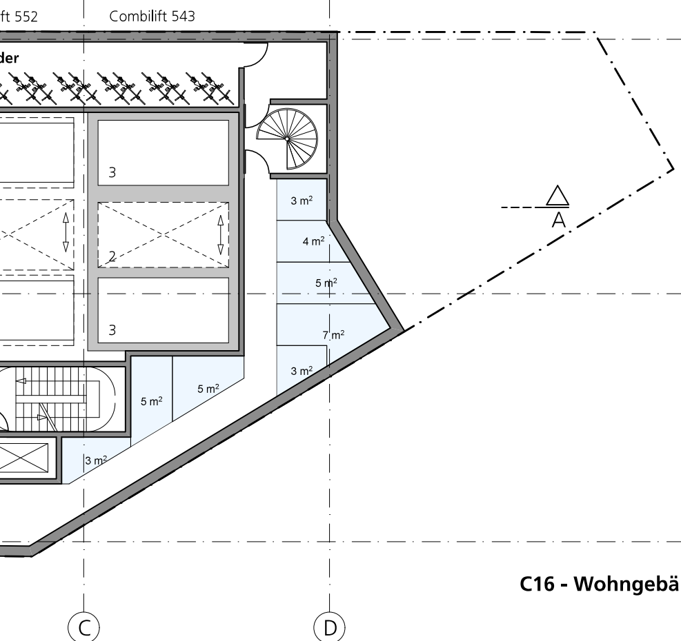
M1:200 (auf Din A3) Grundriss UG Stand: 19.01.2017
